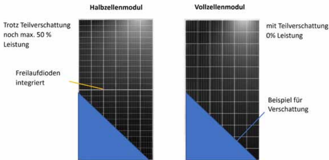
Bild 1: Unterschied zwischen Voll- und Halbzellenmodul beim Einfluss einer Teilverschattung
